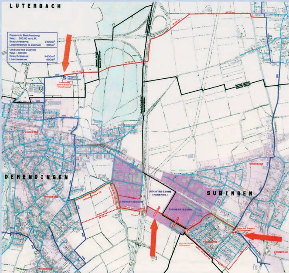
Situationsplan Neue Wasserversorgung ab Derendingen
